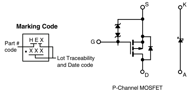
P-Channel MOSFET
